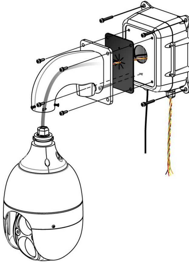
－ スピードドームジャンクションボックスの取り付け －
